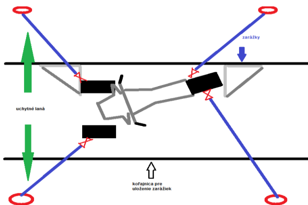
Obr.č.4 - Upevnění tříkolky s jedním kolem vpředu
