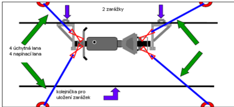
Obr.č.1 - Upevnění motocyklu
